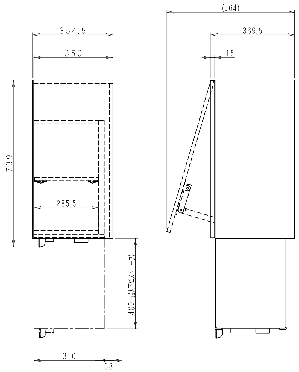
扉取付時寸法 (扉厚み15mm時)
